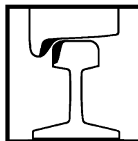
Hjulflänsar
